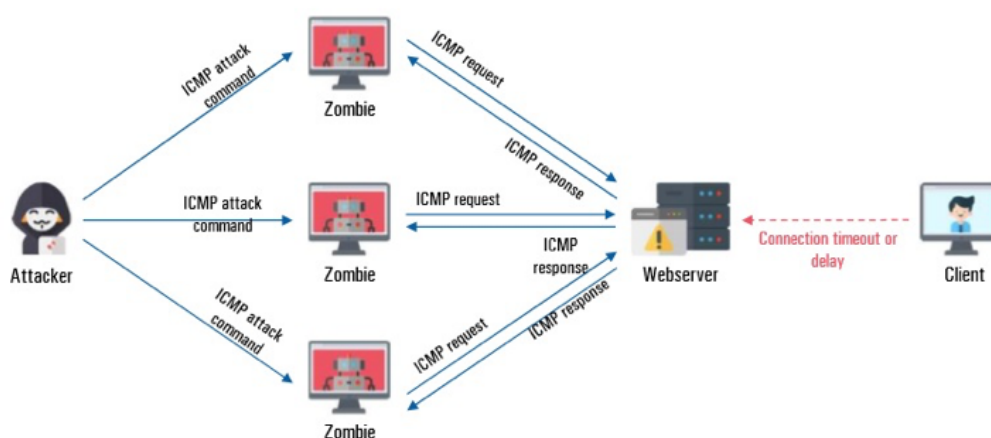
Slika 6 – Standardni ICMP Flood napad
